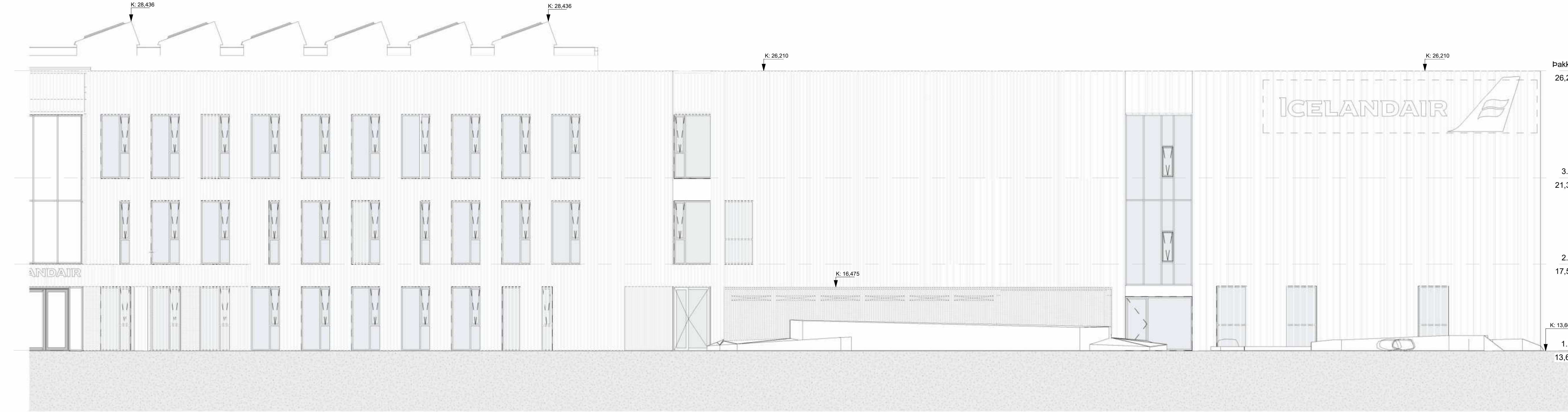
ÚTLIT NORÐUR 1 1:100
